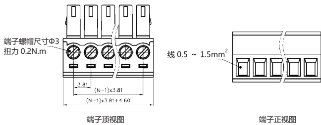
端子接线安装示意图
