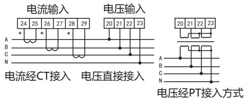
方式1(3个CT):三相四线的接线方式
