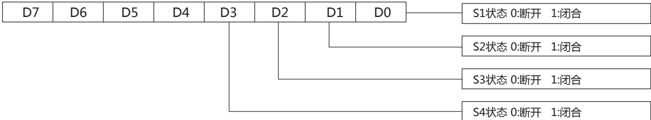
注⑥:测量状态指示 (遥控输入, 通信写0x4a09)
