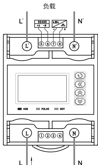
单相两线直接输入 (适用于最大电流80A的仪表)
