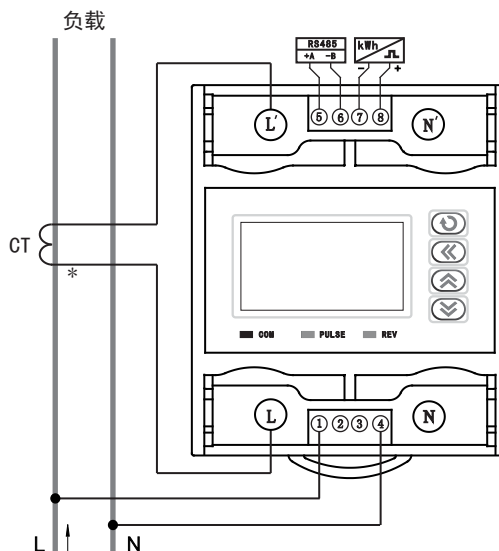
单相两线经电流互感器输入 (适用于最大电流6A的仪表)
