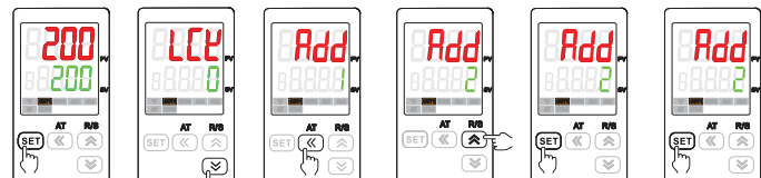
长按“SET”键3秒进入常用菜单 短按“+”或“-”键切换菜单 短按“K”键参数闪烁 短按“+”或“-”键修改参数 短按“SET”键保存参数 长按“SET”键3秒退出菜单
