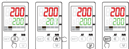
短按“K”键SV值闪烁 短按“+”键增加SV值 短按“-”键减少SV值 短按“SET”键保存SV值
