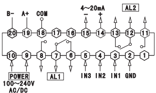
电压输入接线图
