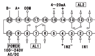
电流输入接线图
